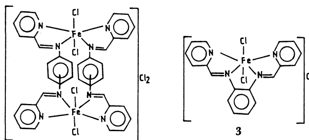
1, Bridge= p -phenylenediamine 2, Bridge= m -phenylenediamine
